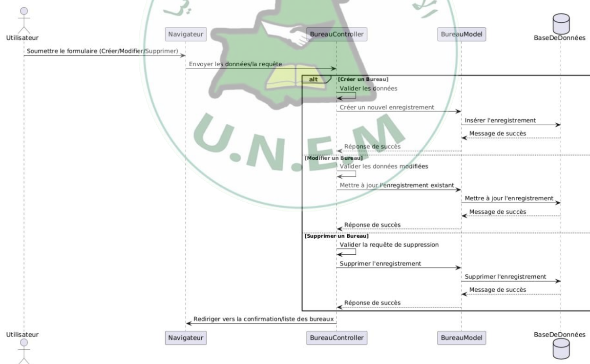
Figure 13: Diagramme de séquence pour les bureaux
